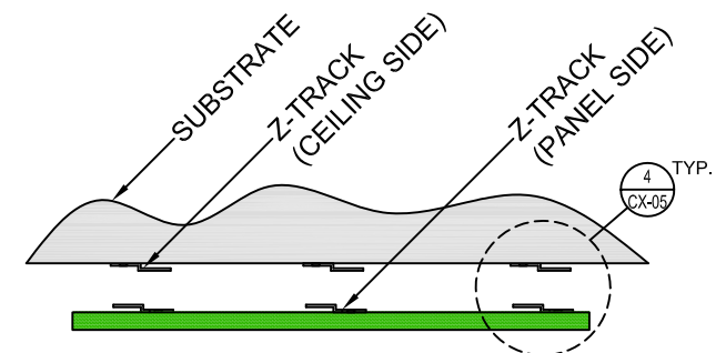
3 CX-05 SIDE VIEW SCALE: NA
